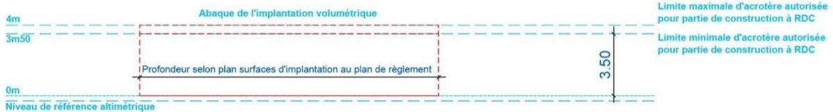
CONSTRUCTION PRINCIPALE, VOLUME EN RDC A TOITURE TERRASSE
