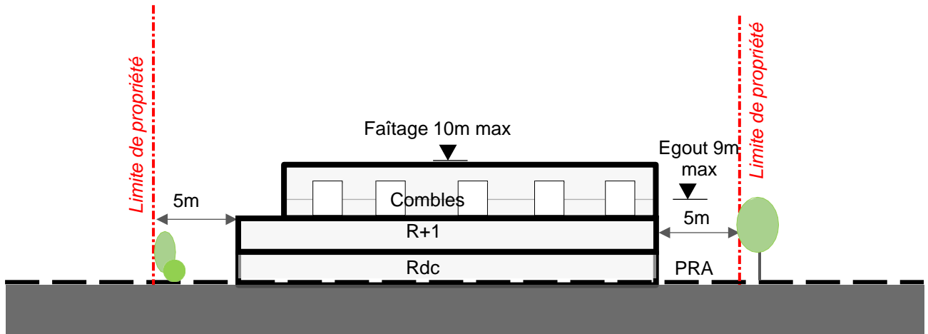
Macrolot 06. Exemple de Coupe longitudinale
