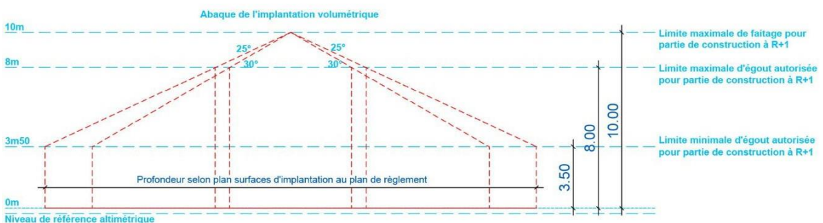
CONSTRUCTION PRINCIPALE, VOLUME EN R+1 OU R+1+COMBLES A TOIT DOUBLE PENTE
