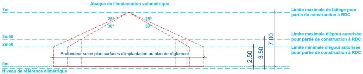
CONSTRUCTION PRINCIPALE, VOLUME EN RDC A TOIT DOUBLE PENTE
