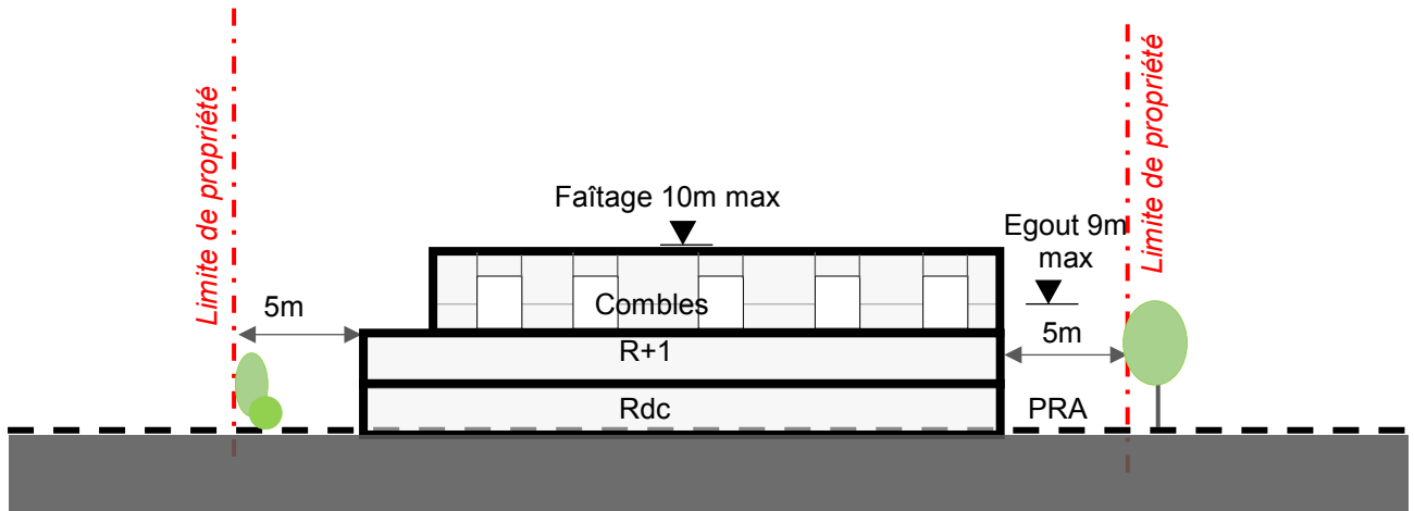
Macrolot 06. Exemple de Coupe longitudinale
