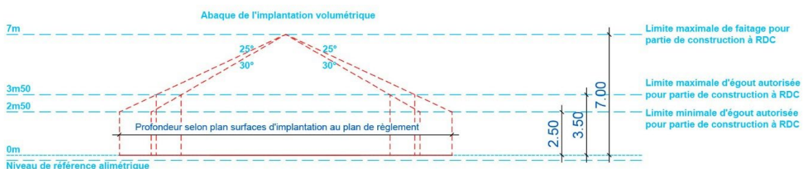
CONSTRUCTION PRINCIPALE, VOLUME EN RDC A TOIT DOUBLE PENTE
